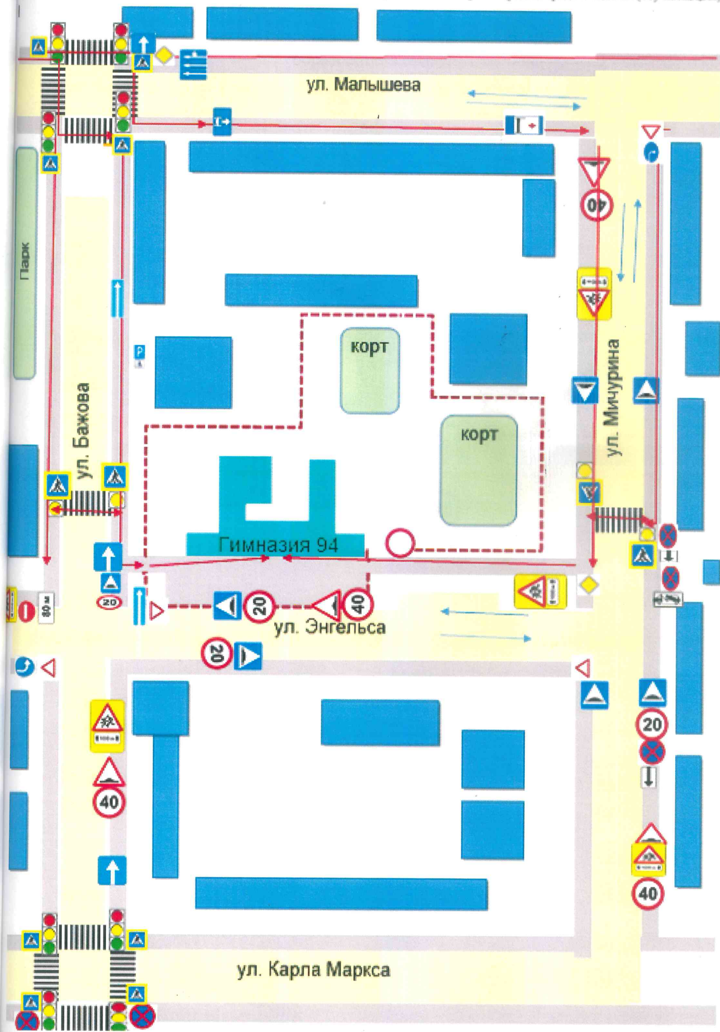
2. Схема организации дорожного движения в непосредственной близости от МАОУ-гимназии №94, с размещением соответствующих технических средств организации дорожного движения, маршрутов движения детей и расположении провозных мест района расположения МАОУ-гимназии №94, пути движения транспортных средств и детей (обучающихся)
